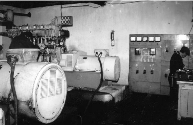
21–22 Dieselmotorkraftwerk, Kovran 1993
